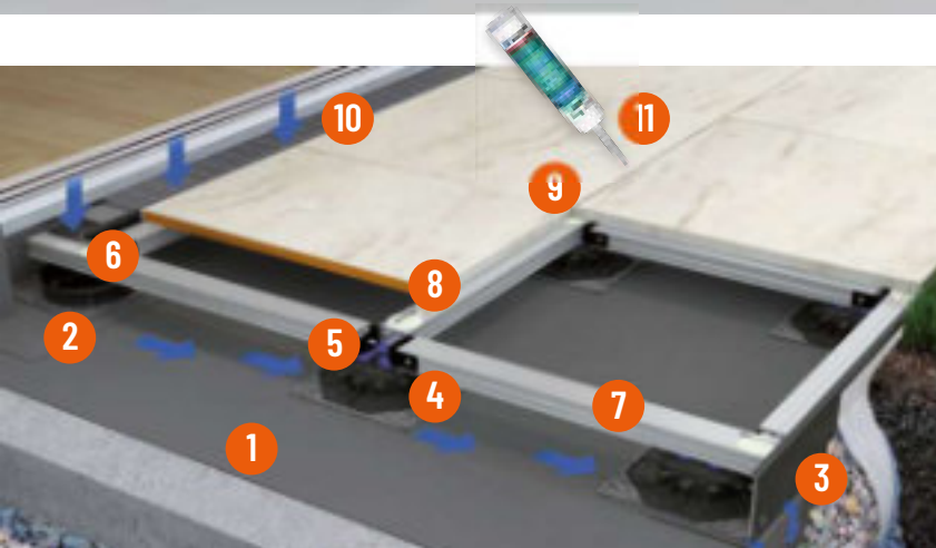
1. DiProtec® KSK Kaltselfstklebebahn, 2. DiProtec® KSK-AB Abdichtungsband, 3. ProFin® KL-H höhenverstellbare Kiesleiste, 4. TerraMaxx® TSL Pad, 5. TerraMaxx® TSL Trockenstetzlager, 6. TerraMaxx® PL Plattenlager, 7. TerraMaxx® RS-S Aluminium-Rahmensystem, 8. TerraMaxx® RS Klebepads, 9. AquaDrain® FF Fugenkreuz, 10. AquaDrain® VARIO Kastenrinne, 11. MorTec® SOFT
