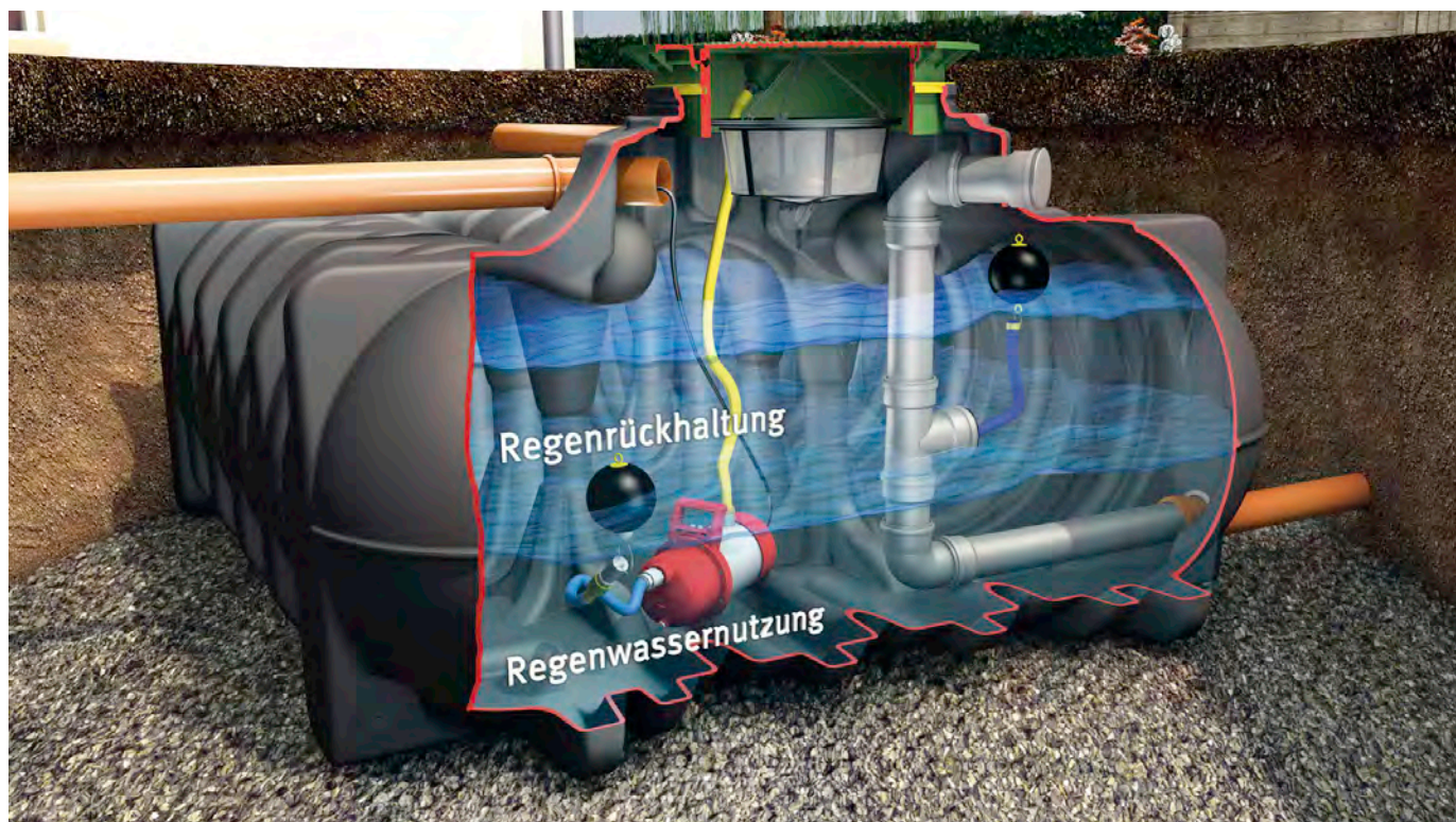
Flachtank Platin Retentionszisterne Plus: Zur kombinierten Regenrückhaltung und Regenwassernutzung.
