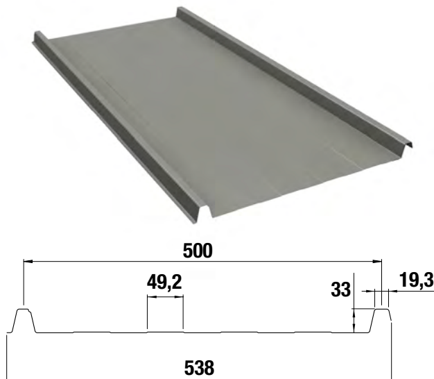
Querschnittszeichnung
