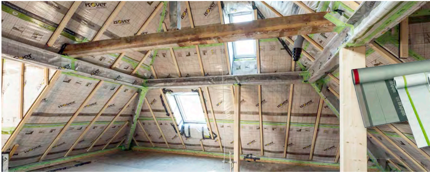
Das Vario® Komplettsystem von ISOVER – alle Komponenten im Überblick
