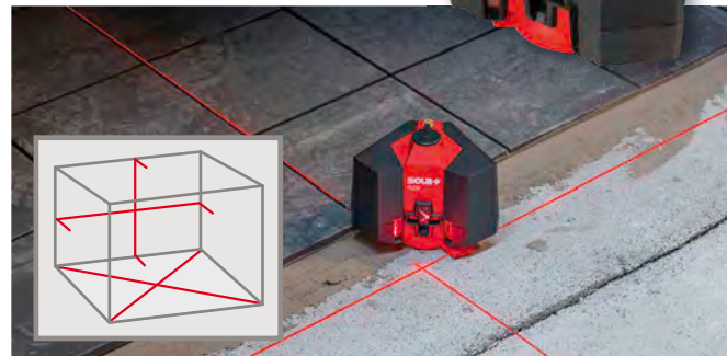
FLOX Boden- und Kreuzlinienlaser
