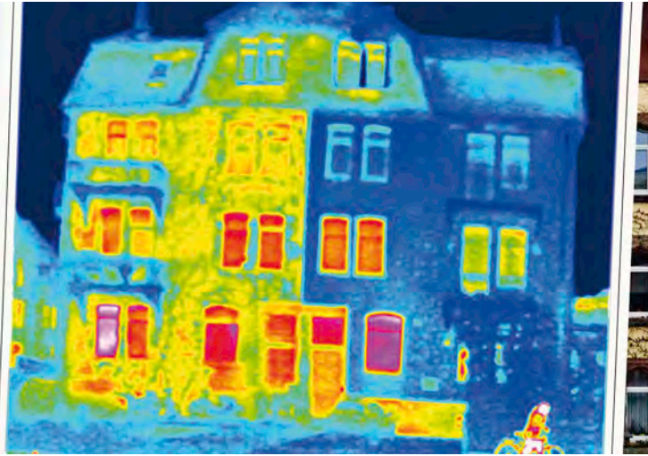
Eine fachgerechte Dämmung erhöht die Wohnqualität und minimiert den Wärmeverlust über die Außenwände.
