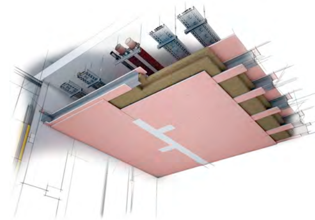
Flamtex A1 Freitragende Unterdecken
