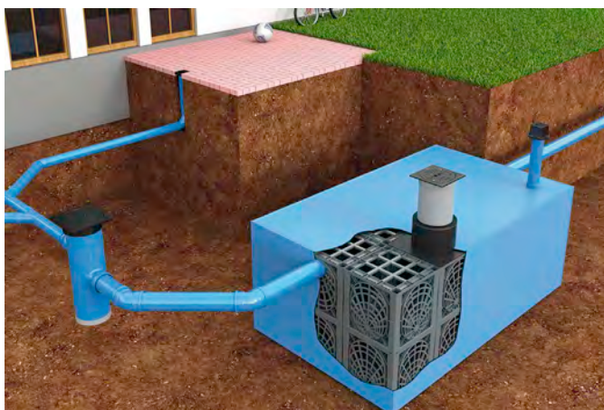
Die KS-Bluebox besteht aus werkseitig mit kunststoffummantelten D-Raintank 3000®-Elementen und dient der Rückhaltung, Speicherung und Nutzung von Regenwasser.
